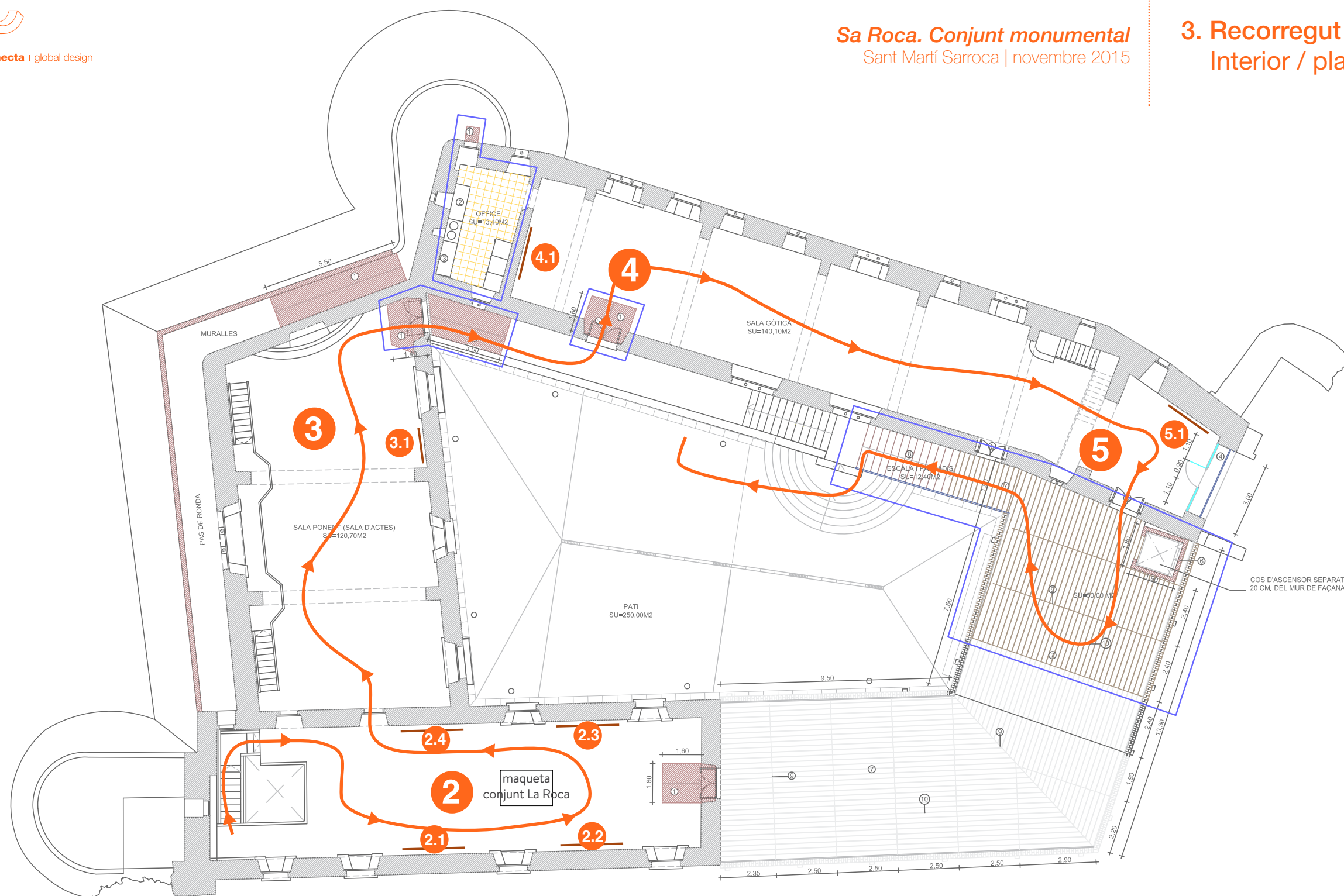
PLANTA NIVELL PL. NOBLE E 1:200
